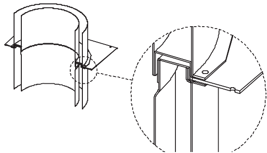
Figure 21 - Section détaillée d'une plaque support
