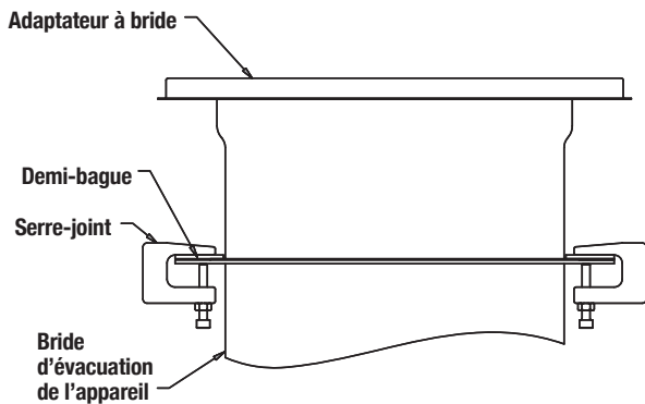
Figure 43 - Adaptateur à bride (FHA illustré)
