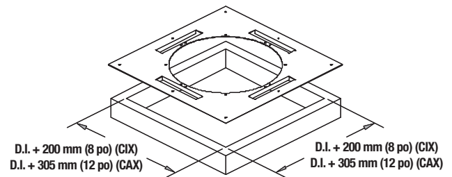
Figure 25 - Plaque de fixation ventilée (APV)
