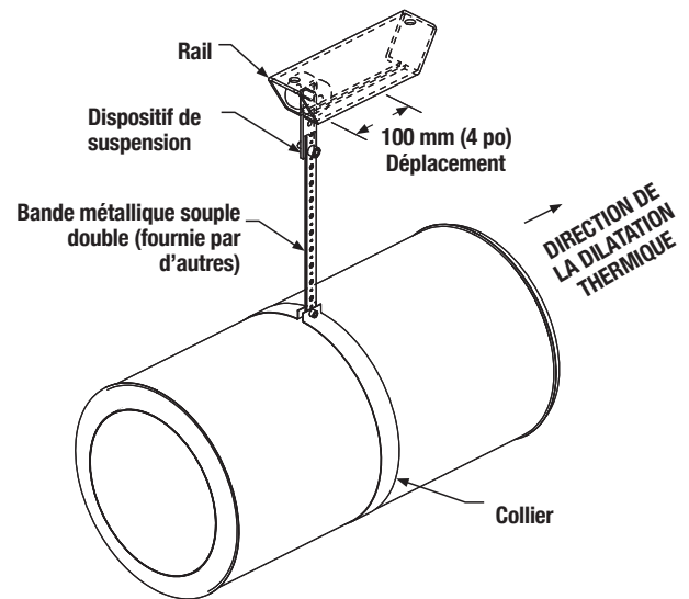
Figure 32 - Dispositif de suspension
