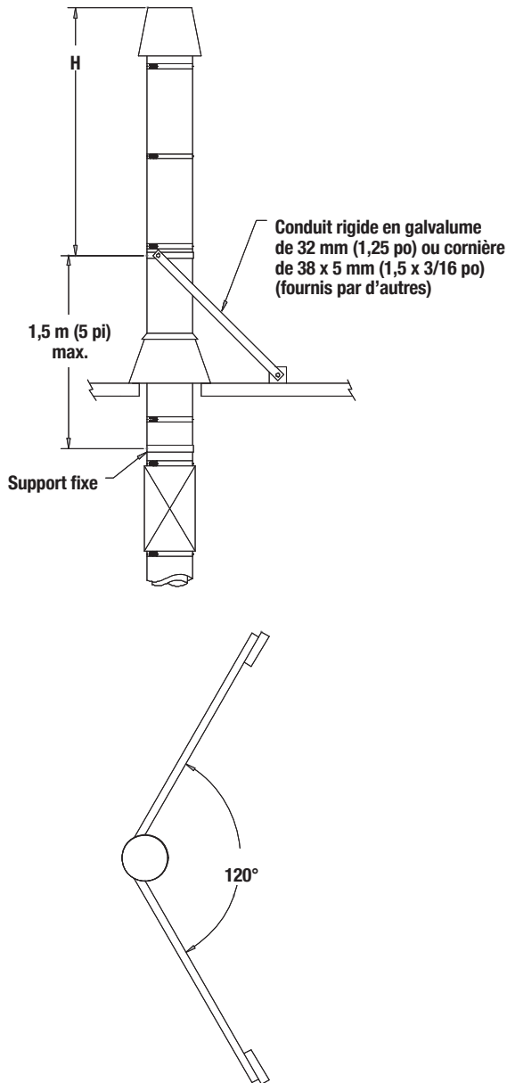
Figure 34 - Ensemble renfort de toit
