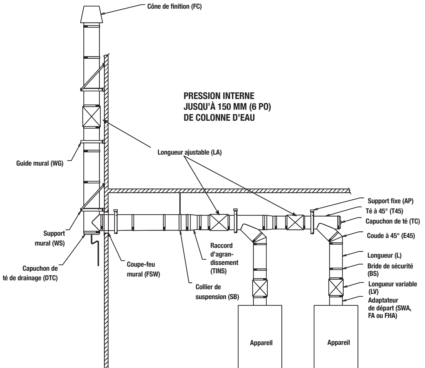
Figure 66 - Emplacement typique d'une longueur ajustable et d'une longueur variable
