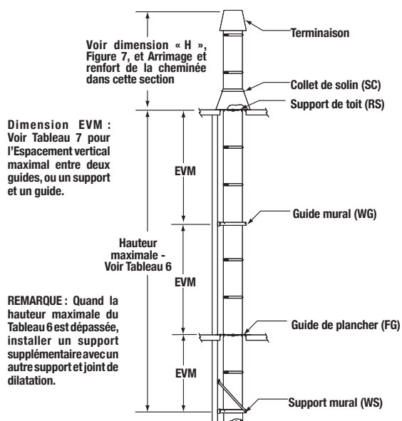
Figure 6 - Support et hauteur maximale de la cheminée
